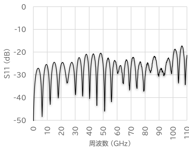
— 反射損失(GSG-150um pitch typ.) —
