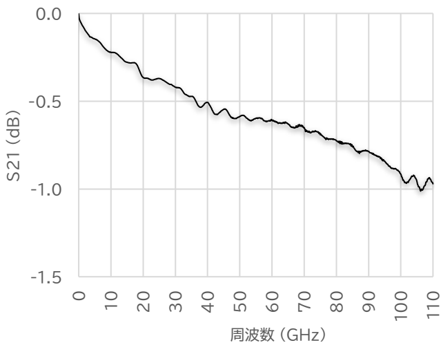
— 挿入損失(GSG-150um pitch typ.) —
